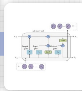
神经网络时代 (LSTM)
